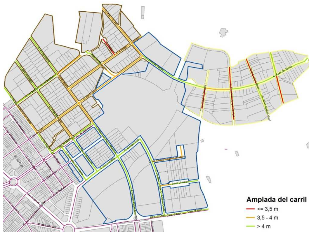
Figura 4.9. Amplada per carril de circulació de les vies del PAE Manlleu
