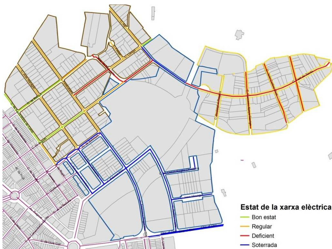
Figura 4.34 Estat de la xarxa elèctrica al PAE Manlleu
