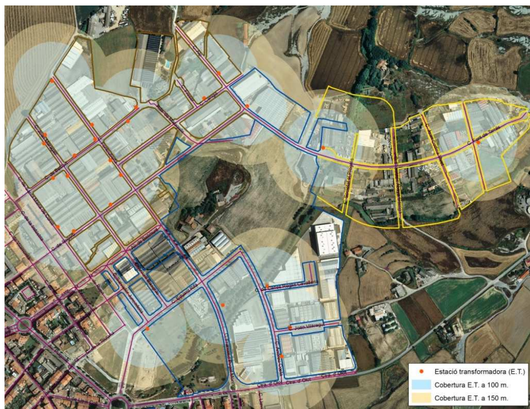
Figura 4.33 Ubicació de les estacions transformadores al PAE Manlleu
