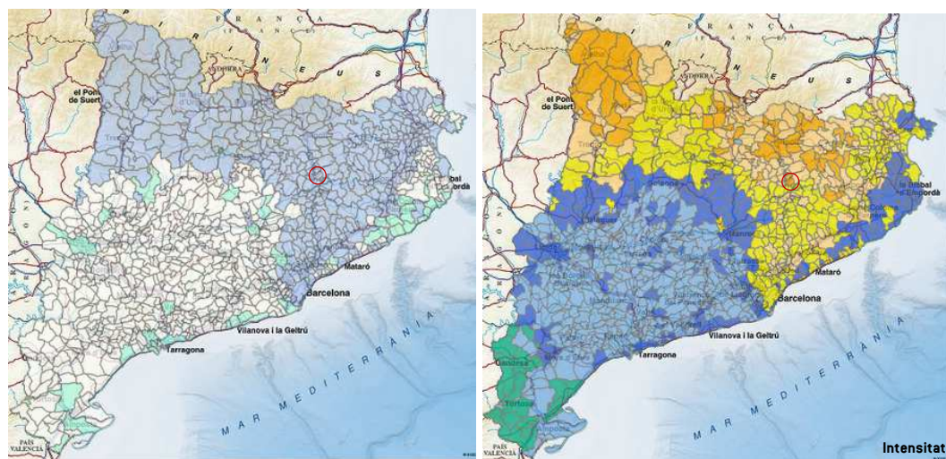
Figura 4.39 Risc sísmic
